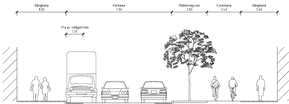
Figur 25 Föreslagen tvärsektion för Leråkersgatan, vy åt nordväst.
